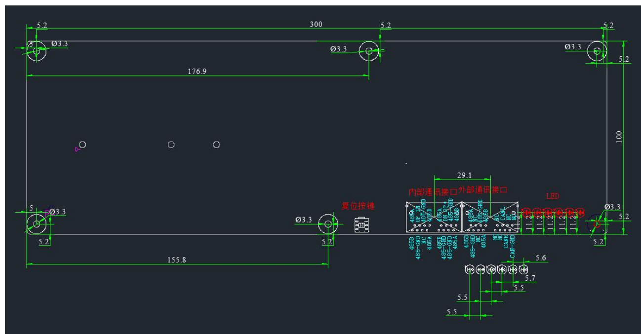
保护板尺寸图: (以结构图为准)
