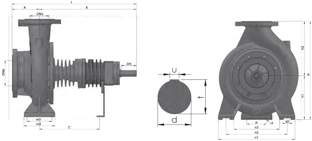
Pompa Ölçüleri / Pump Dimensions (Mm)
