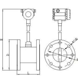
Schemat połączenia kołnierzewego LUGB
