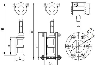
Schemat montażu kołnierza LUGB
