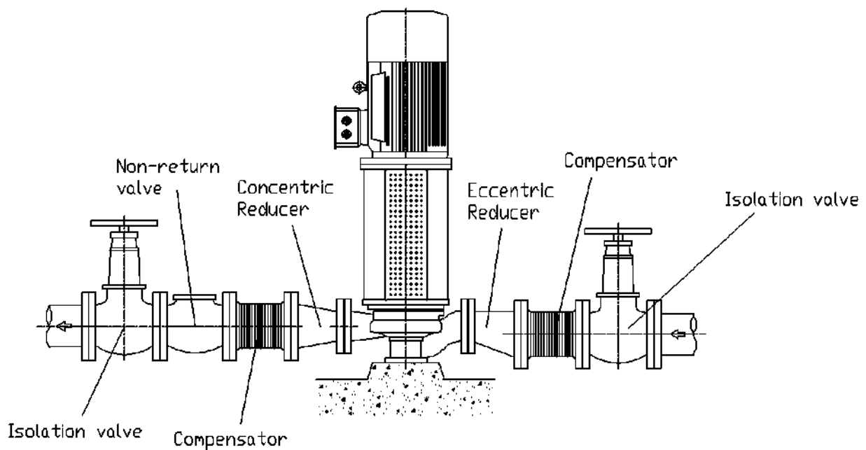
Рисунок 6 підключення трубопроводів
